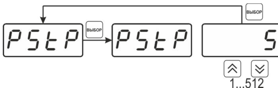
Рисунок 6.34 Задание последнего шага программы
