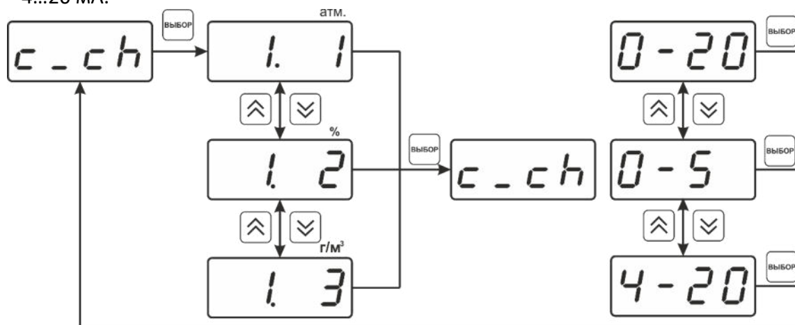
Рисунок 6.23 Настройка входного параметра канала управления (токовый)
