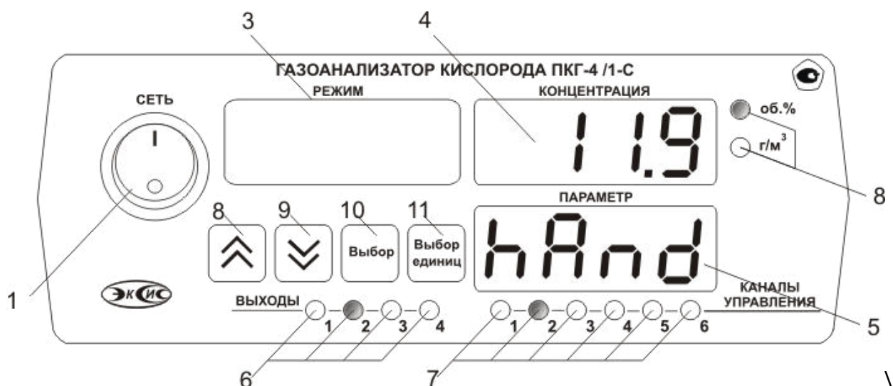
Рисунок 3.2 Вид лицевой панели газоанализатора, исполнение ПКГ-4 /1-С-К-4Р-2А
