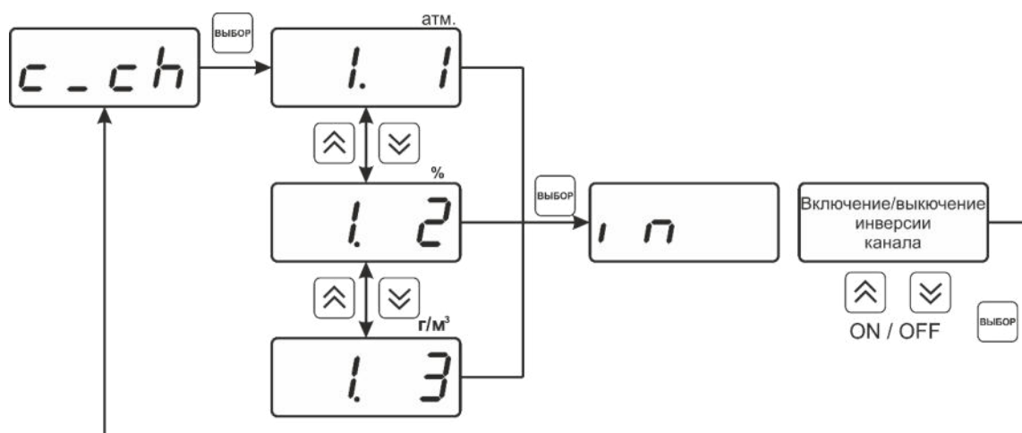
Рисунок 6.22 Настройка входного параметра канала управления (реле)
